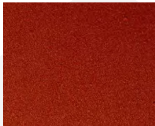
Mars Red
